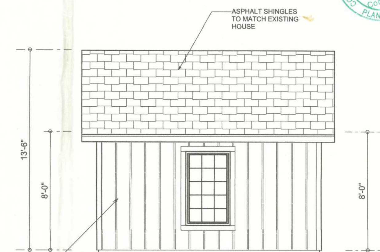
LEFT ELEVATION SCALE: 1/4" = 1'-0"
