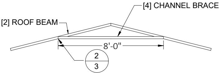
CHANNEL BRACE TRUSS DETAIL SCALE: N.T.S.
