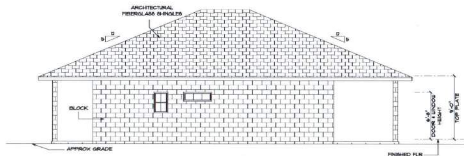
• RIGHT ELEVATION •
