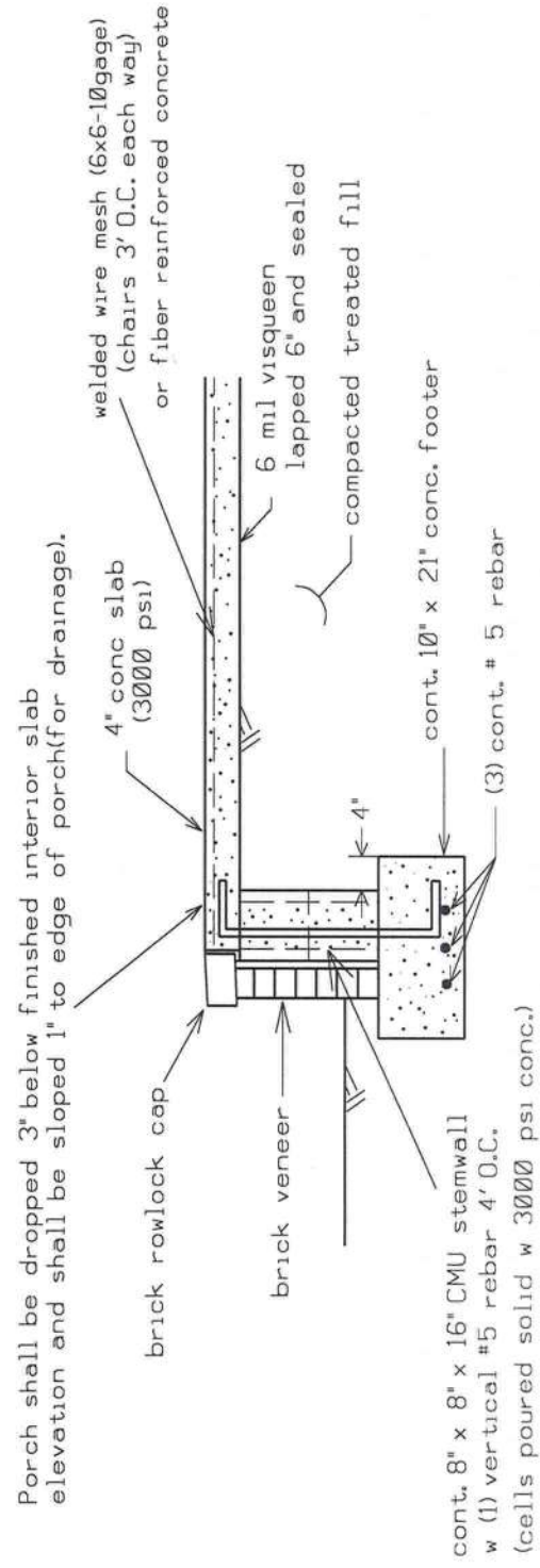
DETAIL B - PORCH FOUNDATION (N.T.S.)
