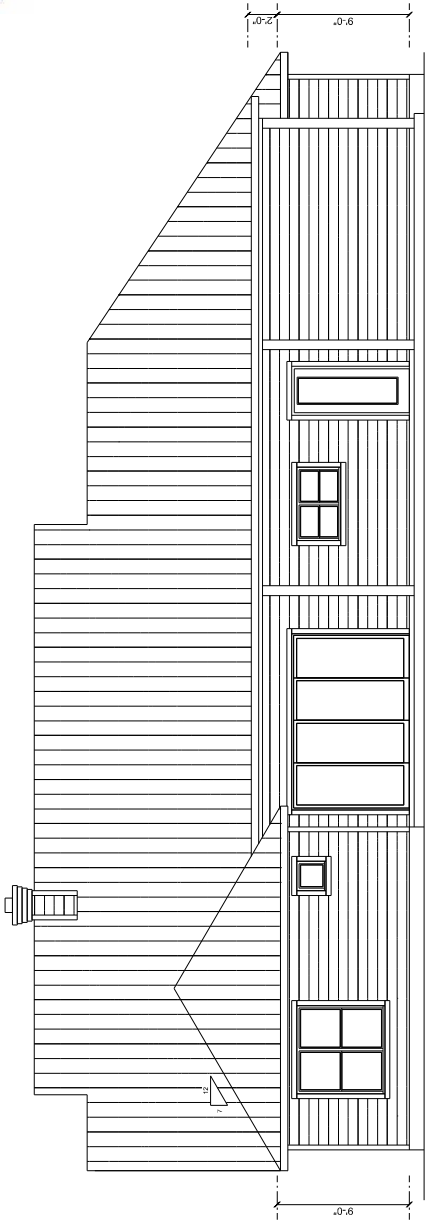
REAR ELEVATION SCALE: 1/8" = 1'-0"
