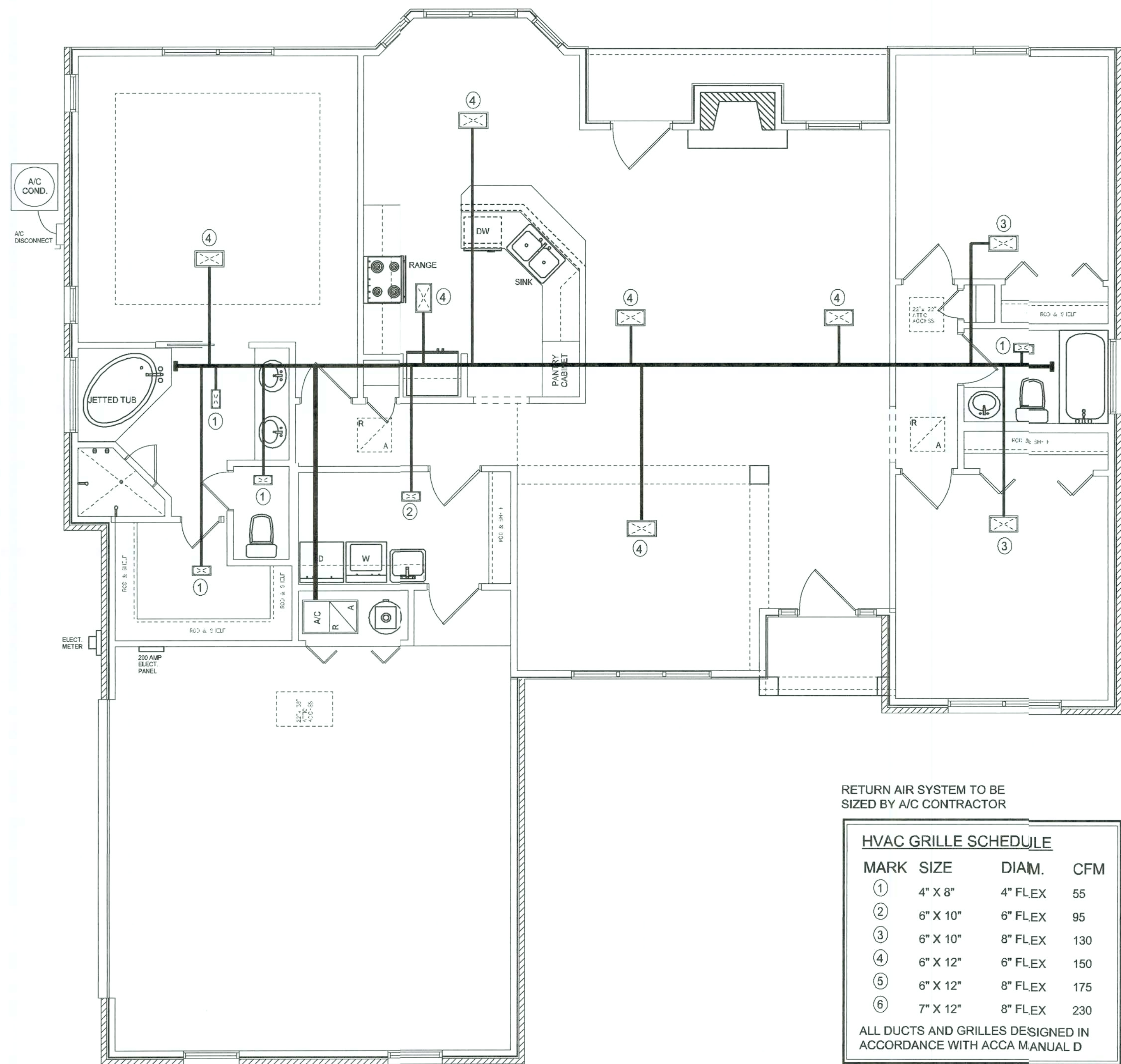
HVAC PLAN SCALE: 1/4" = 1'-0"
