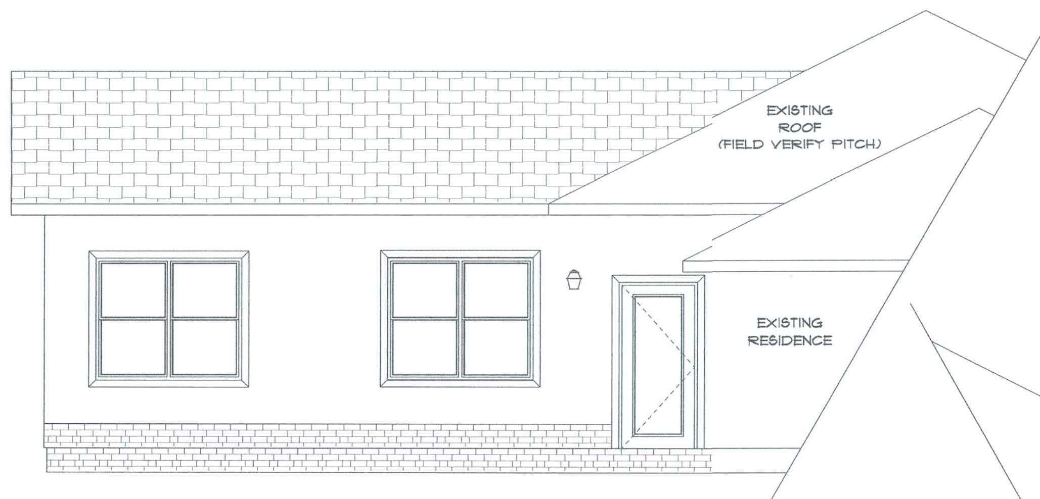
RIGHT ELEVATION
