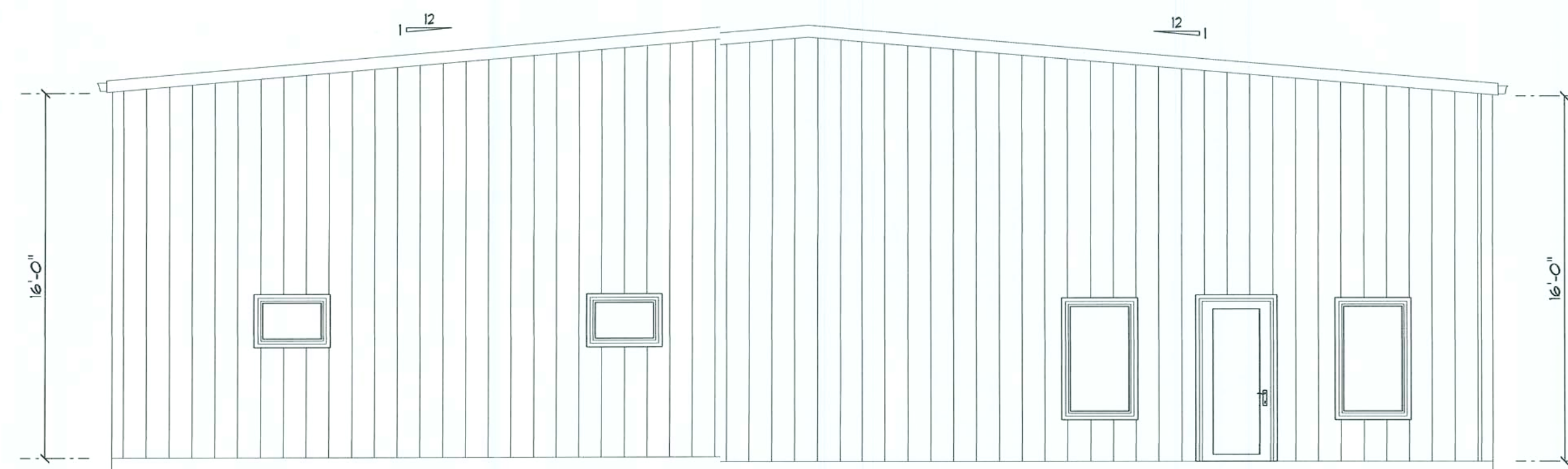
FRONT ELEVATION SCALE: 1/8" = 1'-0"
