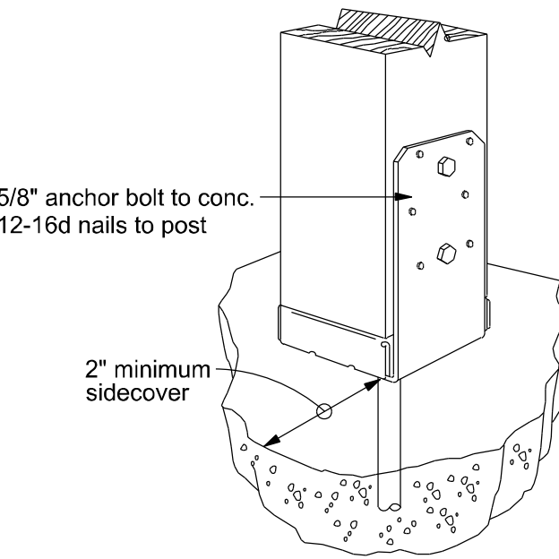
Simpson ABU66
