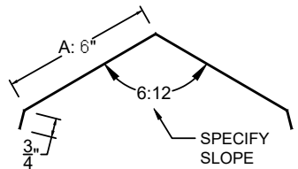
NOTCHABLE CAP (13.5")
