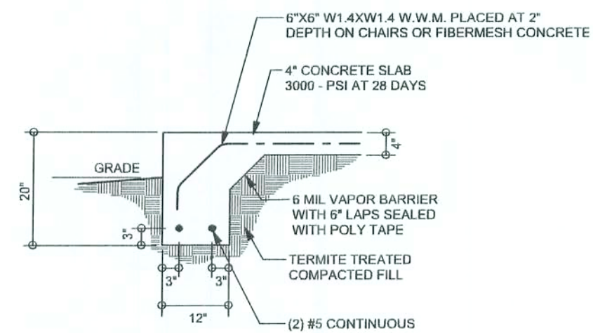
F1 MONOLITHIC FOOTING
