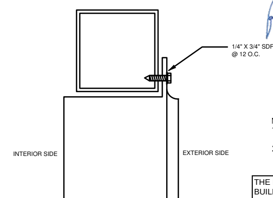
A SECTION SCALE: NTS
