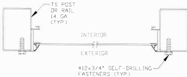
SECTION 2 SCALE: 3"=1'-0"
