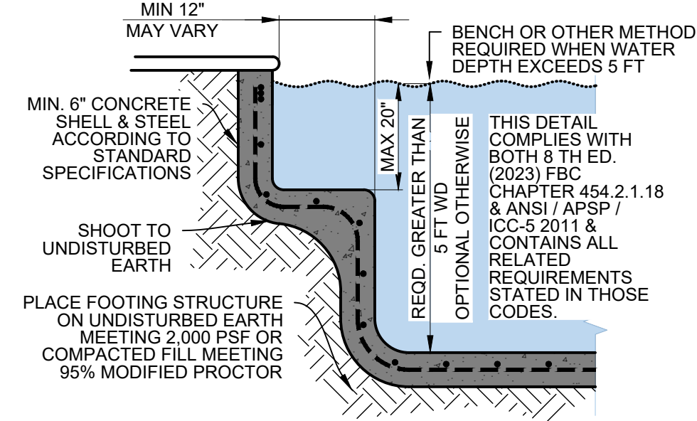
3 BENCH SECTION SCALE: N.T.S.
