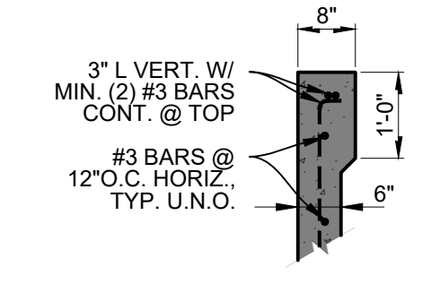
5 POOL BEAM 8"x12" OPTION SCALE: N.T.S.
