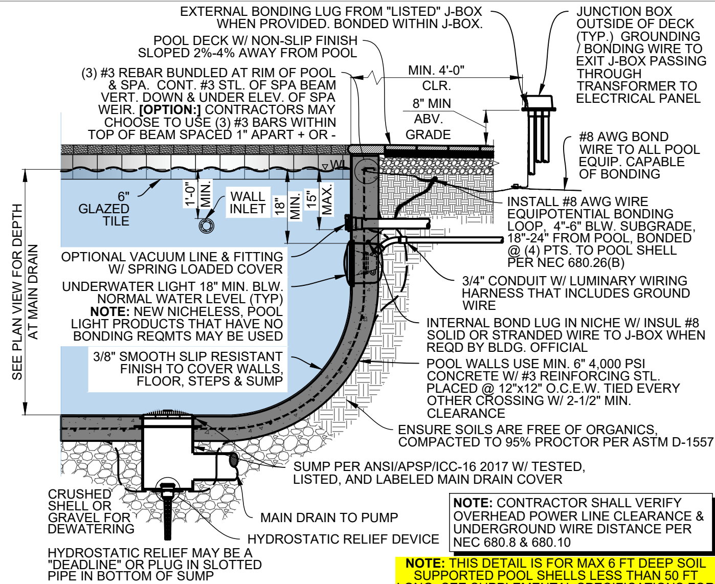
1 POOL DEEP END SECTION SCALE: N.T.S.
