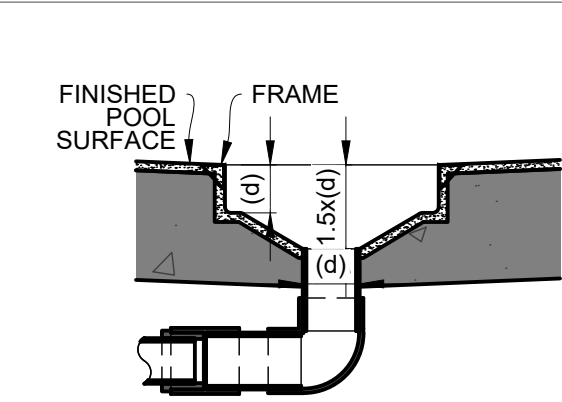
2 FIELD BUILT SUMP SCALE: N.T.S.
