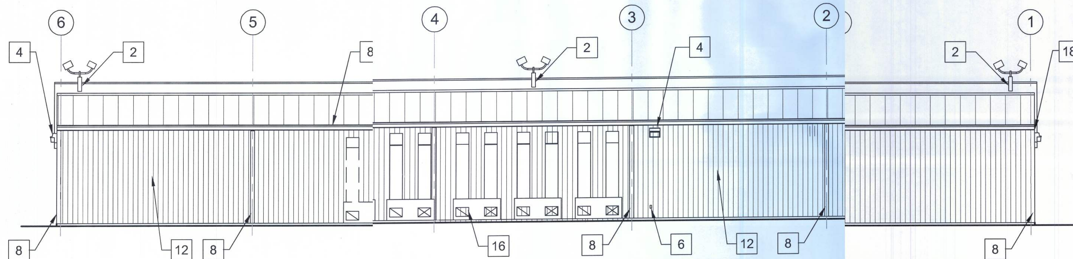
4 REAR ELEVATION A2.C N.T.S.
