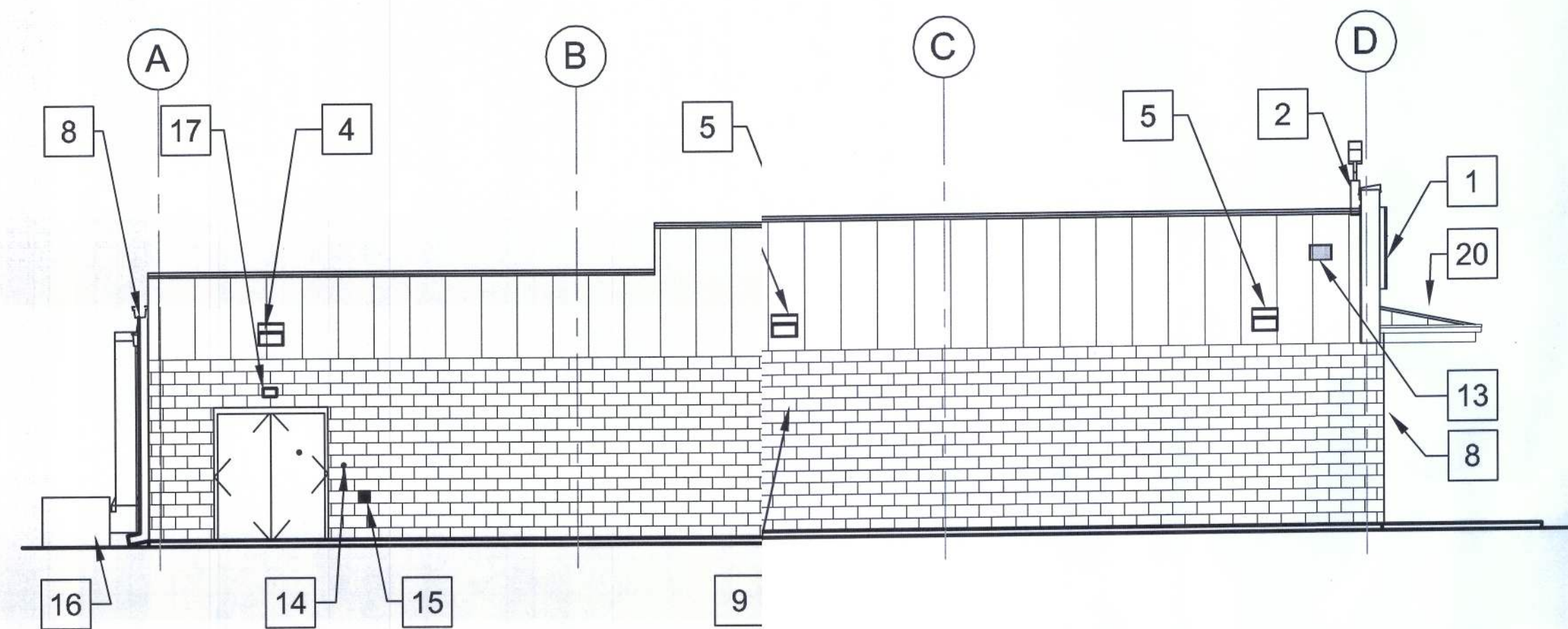
1 LEFT ELEVATION A2.C N.T.S.
