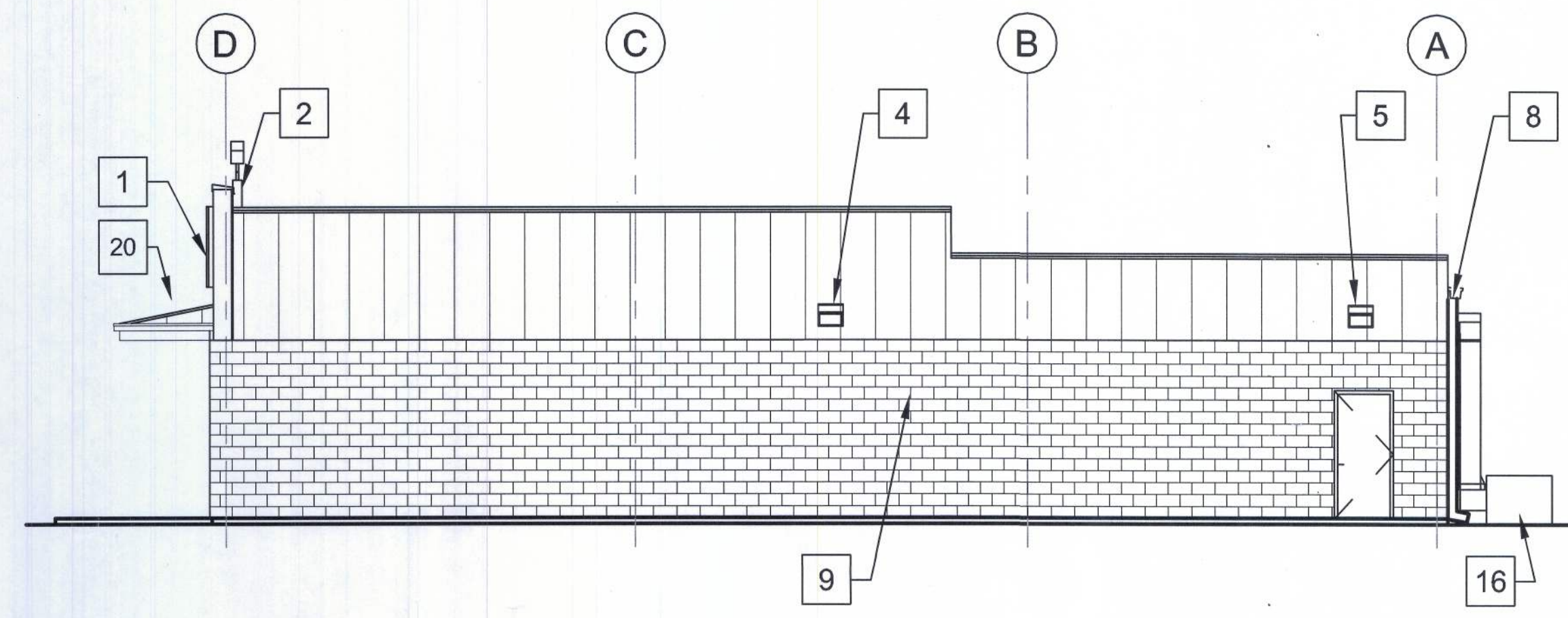
2 RIGHT ELEVATION A2.C N.T.S.
