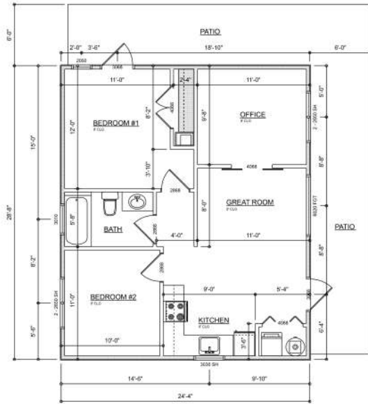
DIMENSIONED FLOOR PLAN SCALE: 1/8" = 1'-0"
