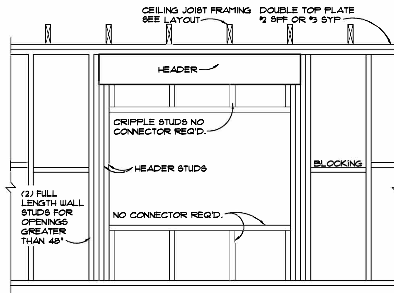
1 Bearing Opening Wood Frame SCALE: N.T.S. NO "UPLIFT"
