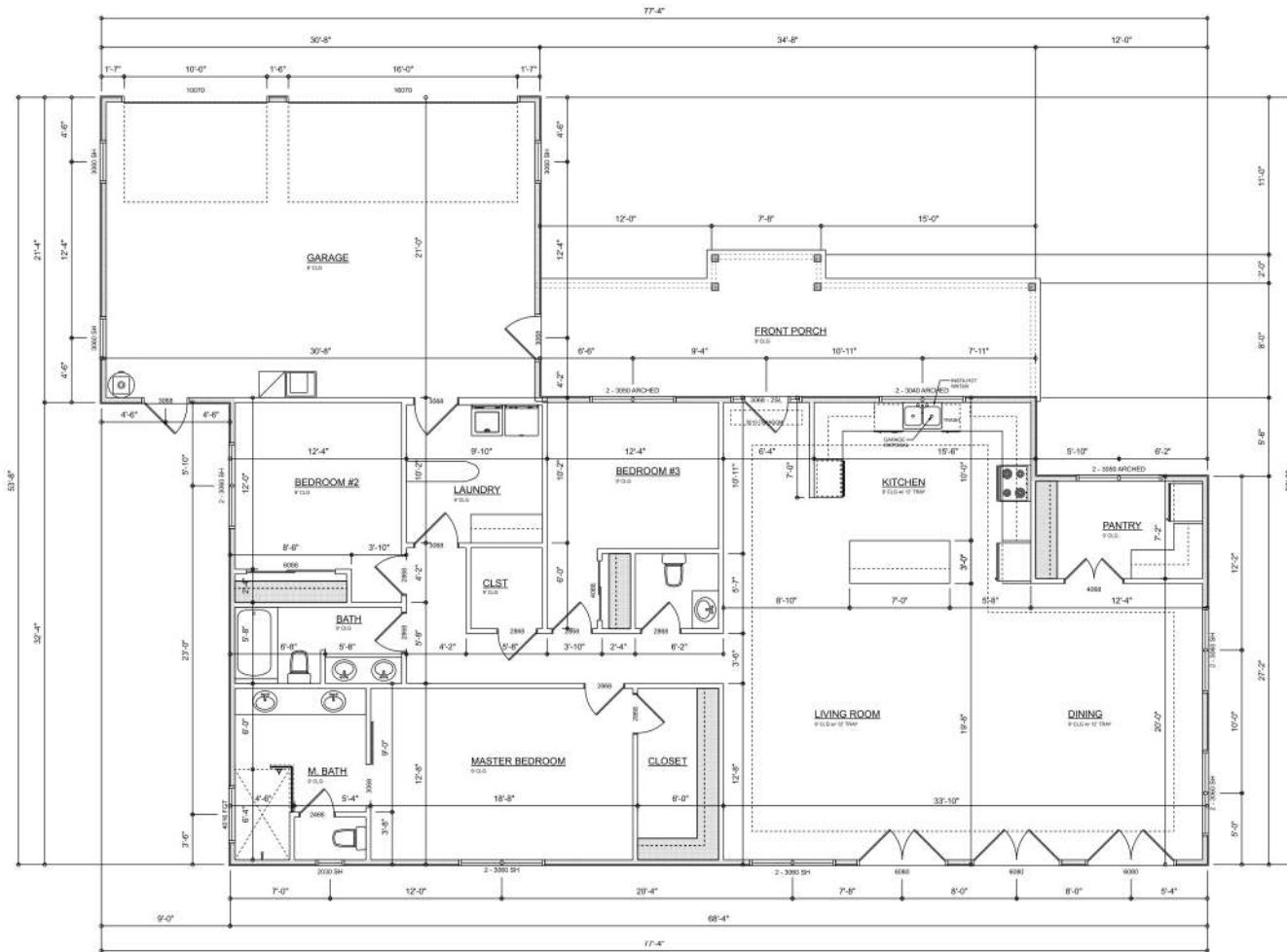
DIMENSIONED FLOOR PLAN SCALE: 1/8" = 1'-0"
