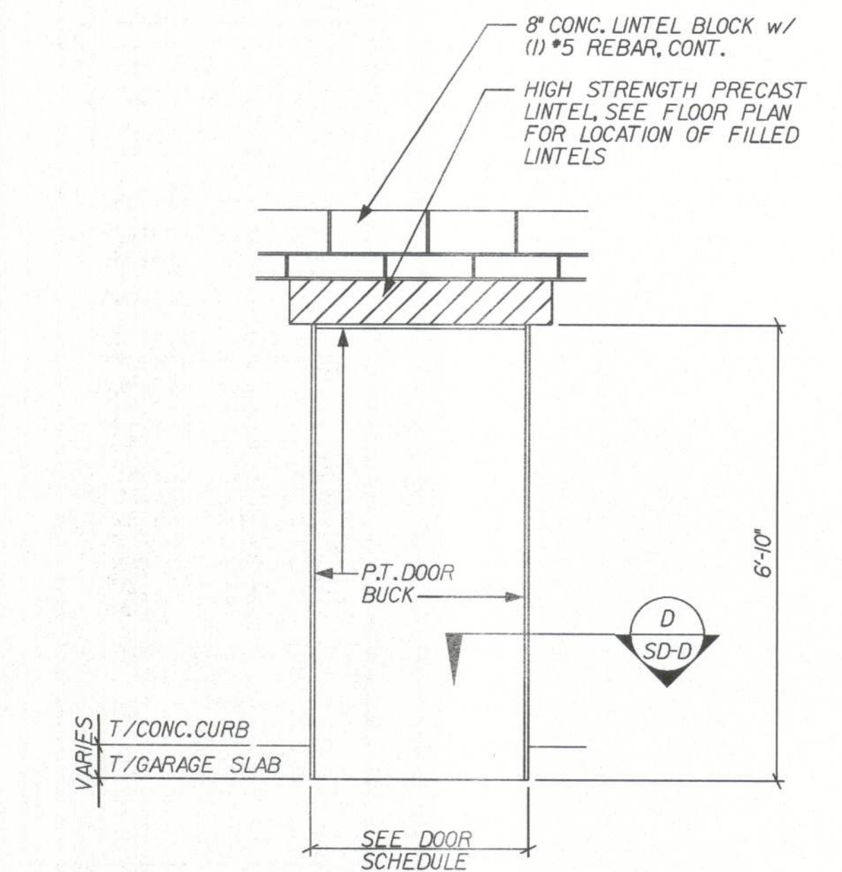
OPTIONAL SERVICE DOOR
