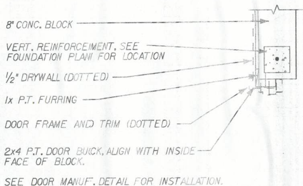
2x DOOR BUCK DETAIL
