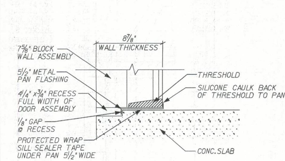
DOOR PAN FLASHING
