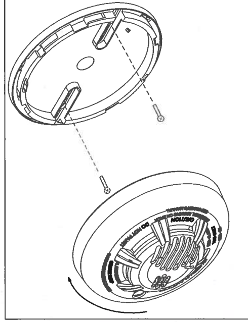
Fig 3. Installation du détecteur
