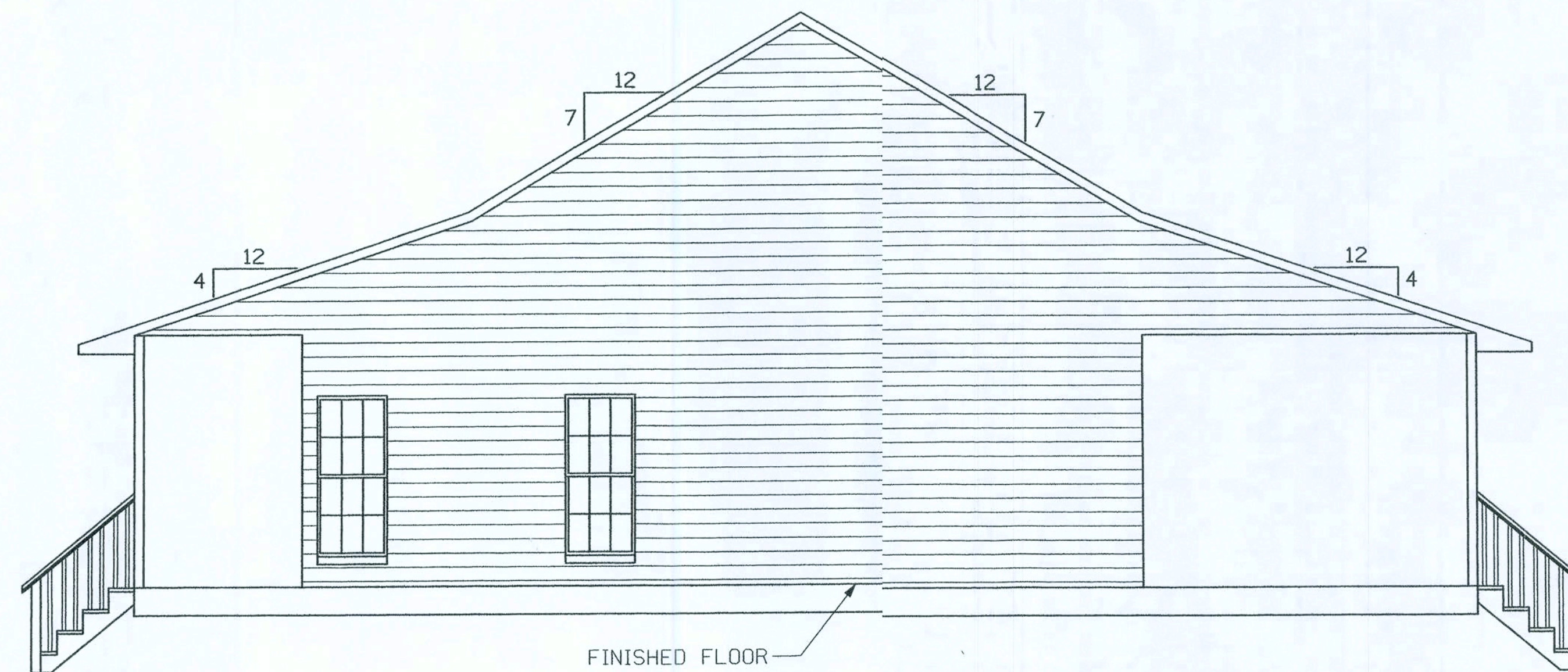
RIGHT ELEVATION
