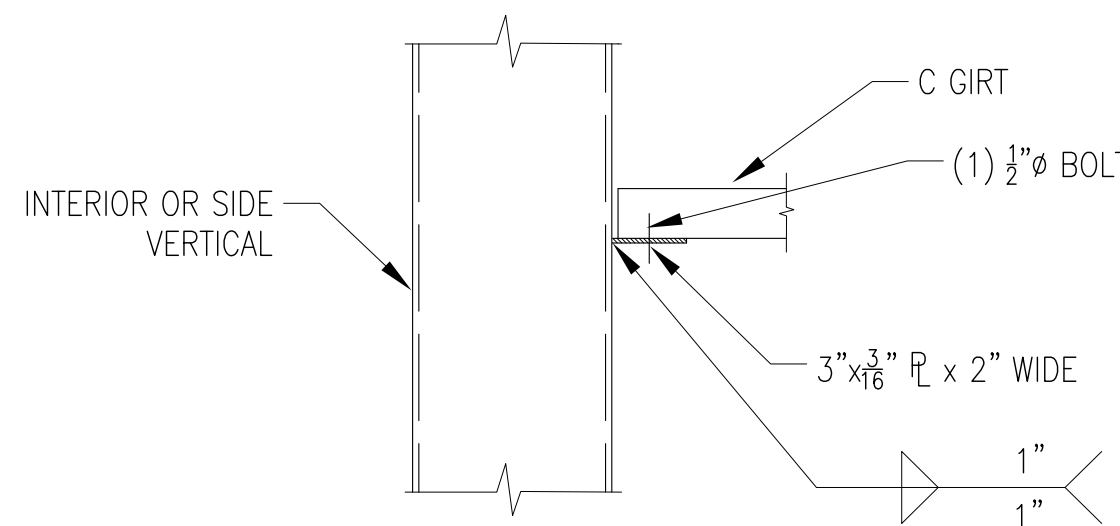
L C GIRT TO VERTICAL Scale: N.T.S.
