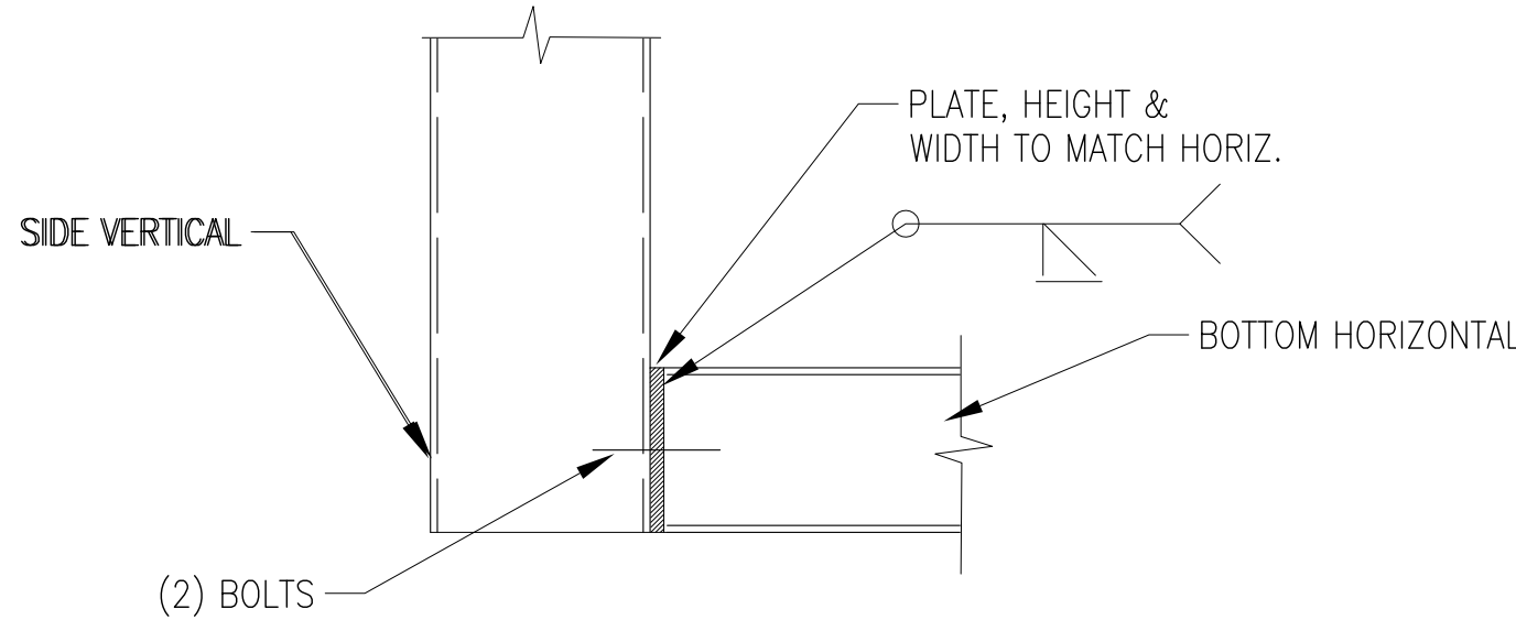
C BOTTOM HORIZONTAL - SIDE VERTICAL Scale: N.T.S.
