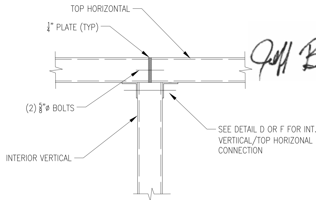
I TOP HORIZONTAL SPLICE - NO SAG TRUSS REQUIRED FOR DOOR WIDTH >53' Scale: N.T.S.
