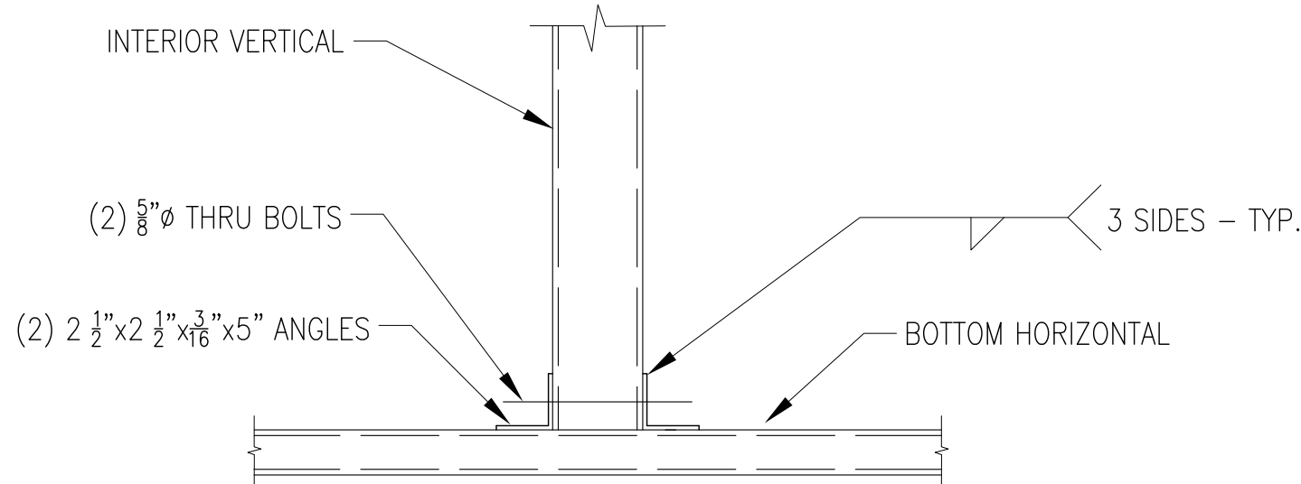
G 6"+ INTERIOR VERTICAL - BOTTOM HORIZONTAL Scale: N.T.S.
