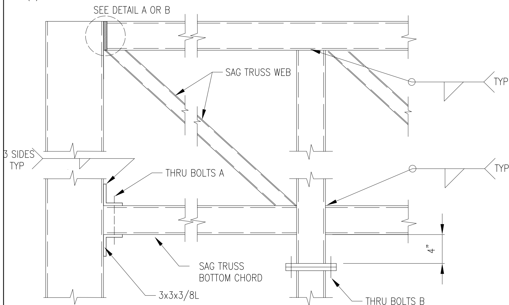
H SAG TRUSS Scale: N.T.S.
