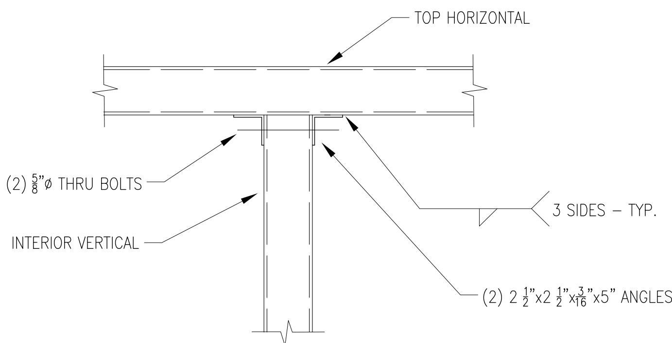
F 6"+ INTERIOR VERTICAL - TOP HORIZONTAL Scale: N.T.S.
