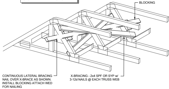
TB02 CROSS BRACING TYPICAL SCALE: N.T.S.
