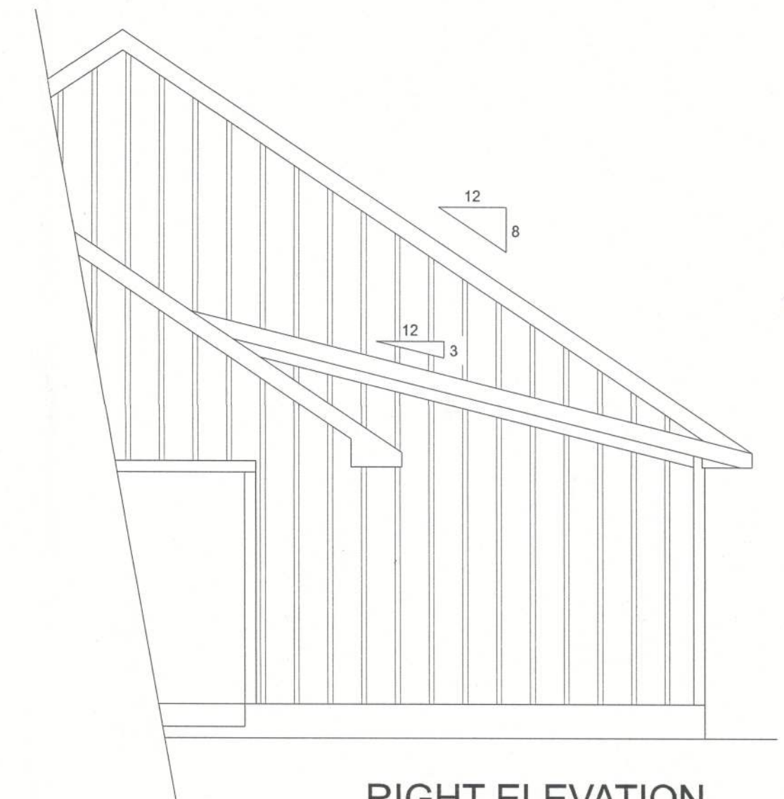
RIGHT ELEVATION SCALE: 1/4" = 1'-0"
