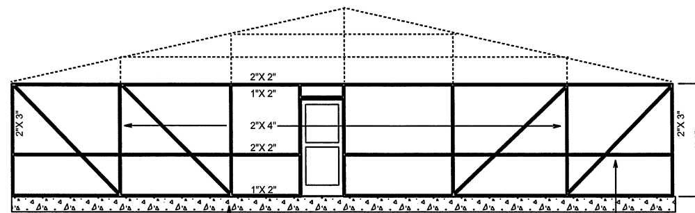
ELEVATION
