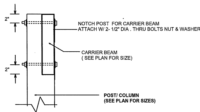
POST/ COLUMN TO BEAM N.T.S.
