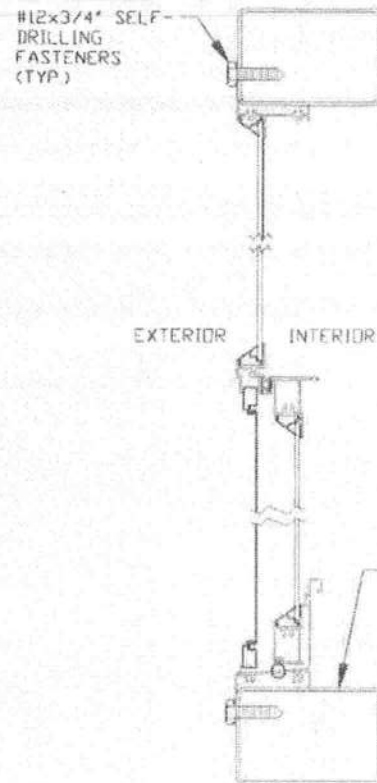
SECTION 1 SCALE: 3"=1'-0"
