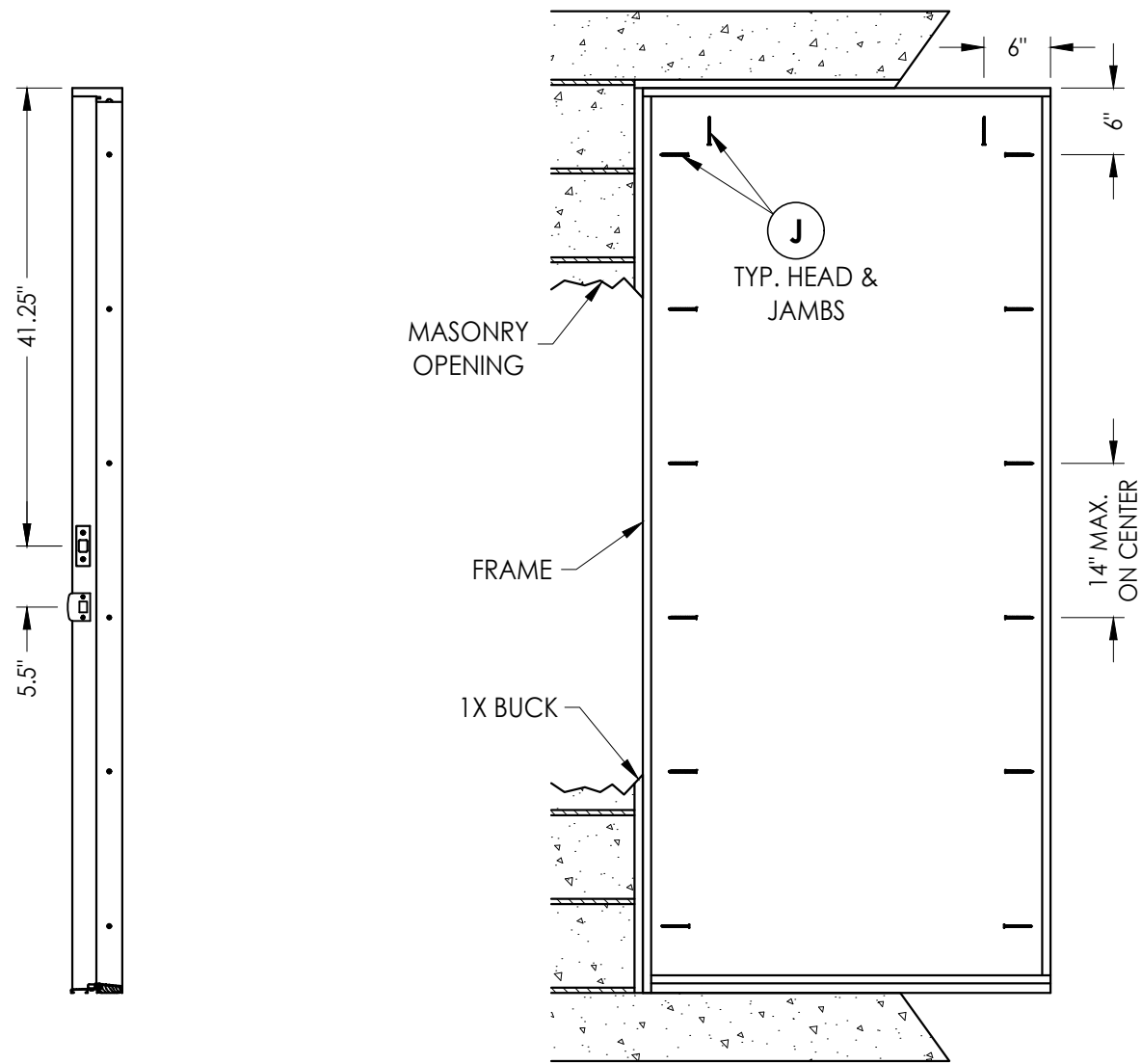
STRIKE JAMB
