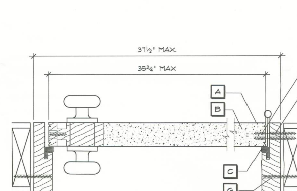
HORIZONTAL SECTION - SINGLE DOOR
