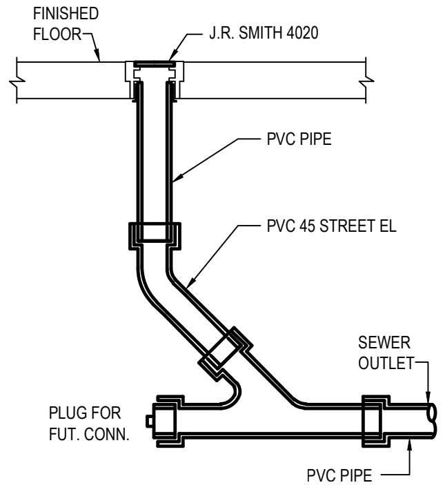
16 | INTERIOR CLEANOUT DETAIL N.T.S.
