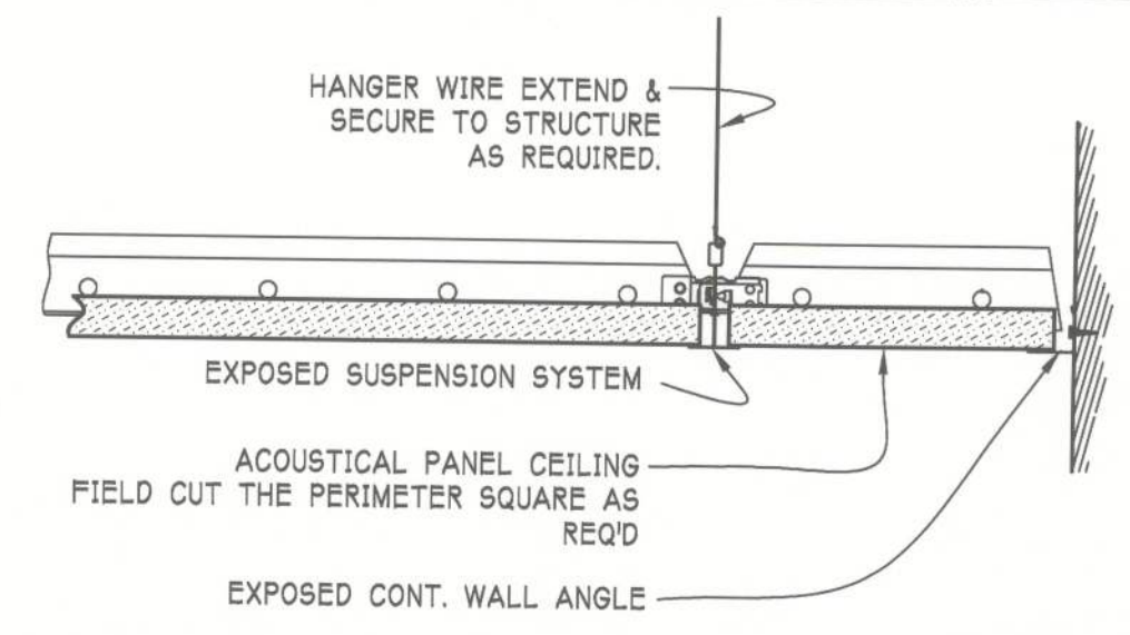
5A APC DETAIL (TYP.) A6.1 SCALE: 3" = 1'-0"
