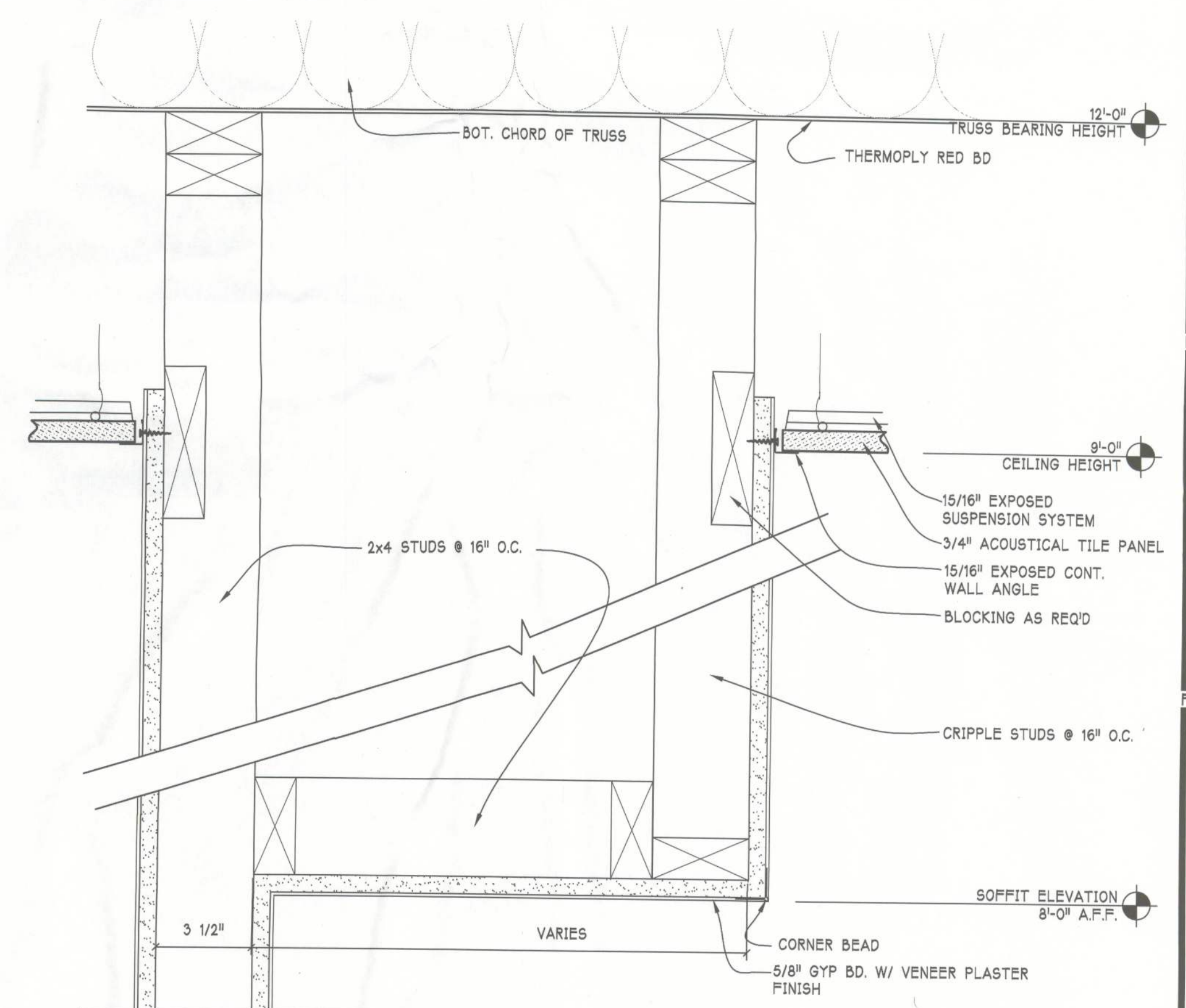
7G SOFFIT DTL A6.1 SCALE: 3" = 1'-0"
