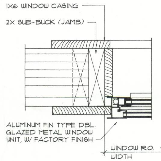
JAMB DETAILS MTL. SASH
