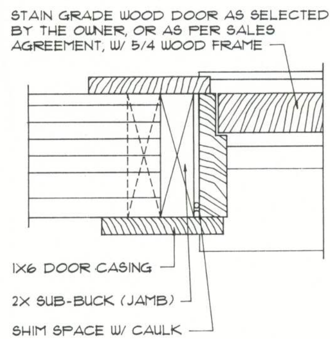
JAMB DETAIL DOOR
