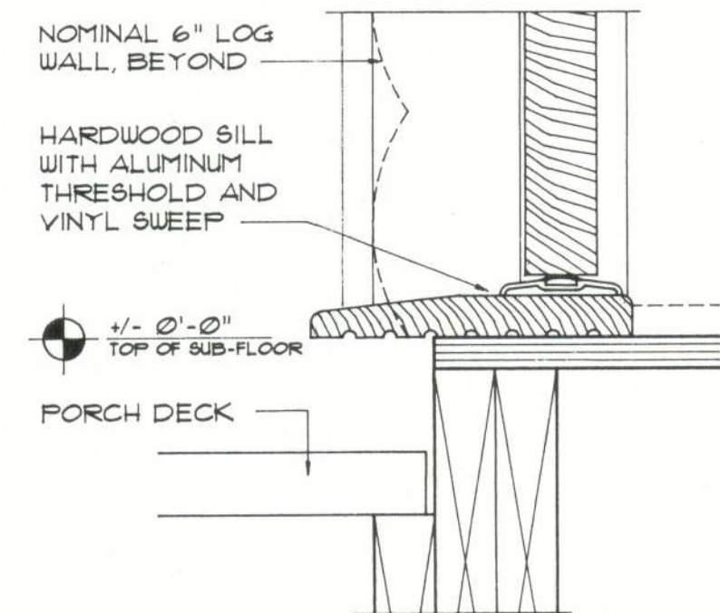
SILL DETAIL DOOR
