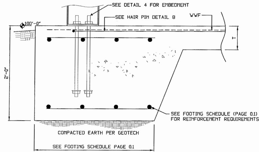
DETAIL 1A
