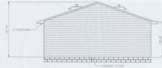
RIGHT ELEVATION
