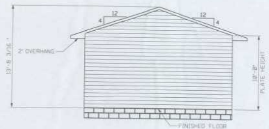
RIGHT ELEVATION
