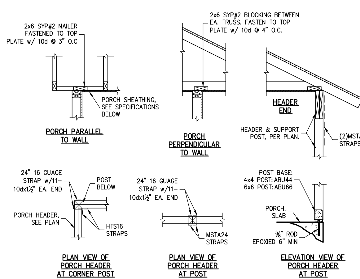
2 TYPICAL PORCH FRAMING DETAILS S.O.1 SCALE: N.T.S.
