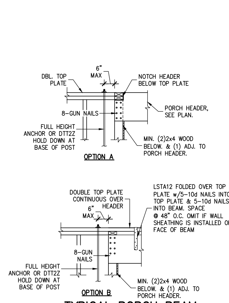
3 TYPICAL PORCH BEAM CONNECTION S.O.1 SCALE: N.T.S.
