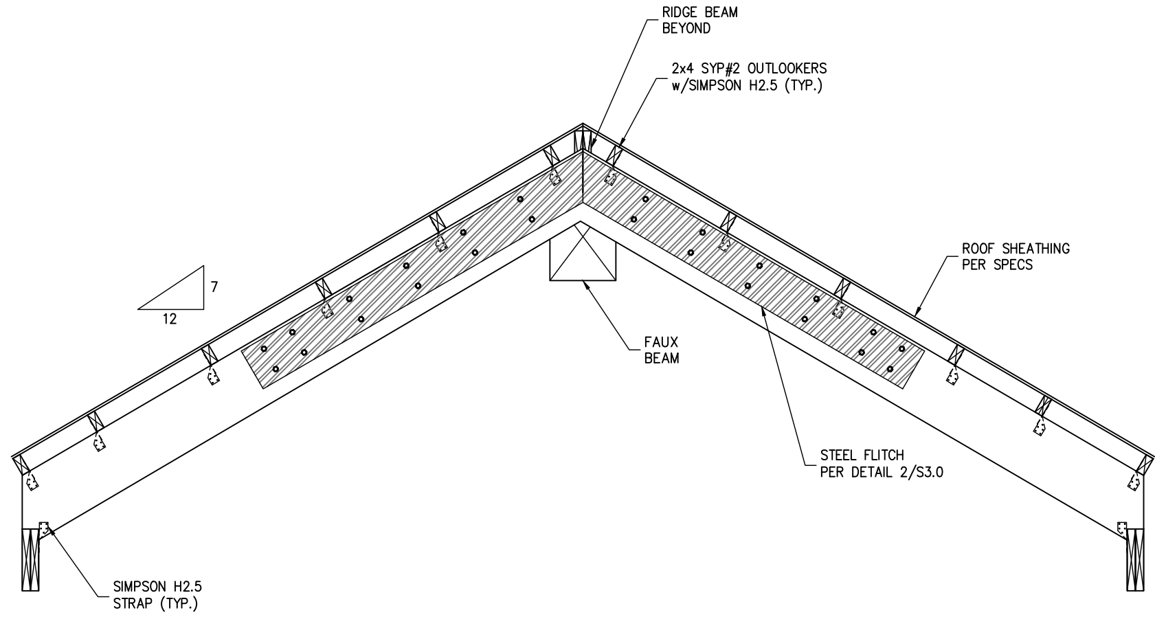
1 ROOF ELEVATION AT ENTRY SCALE: N.T.S.
