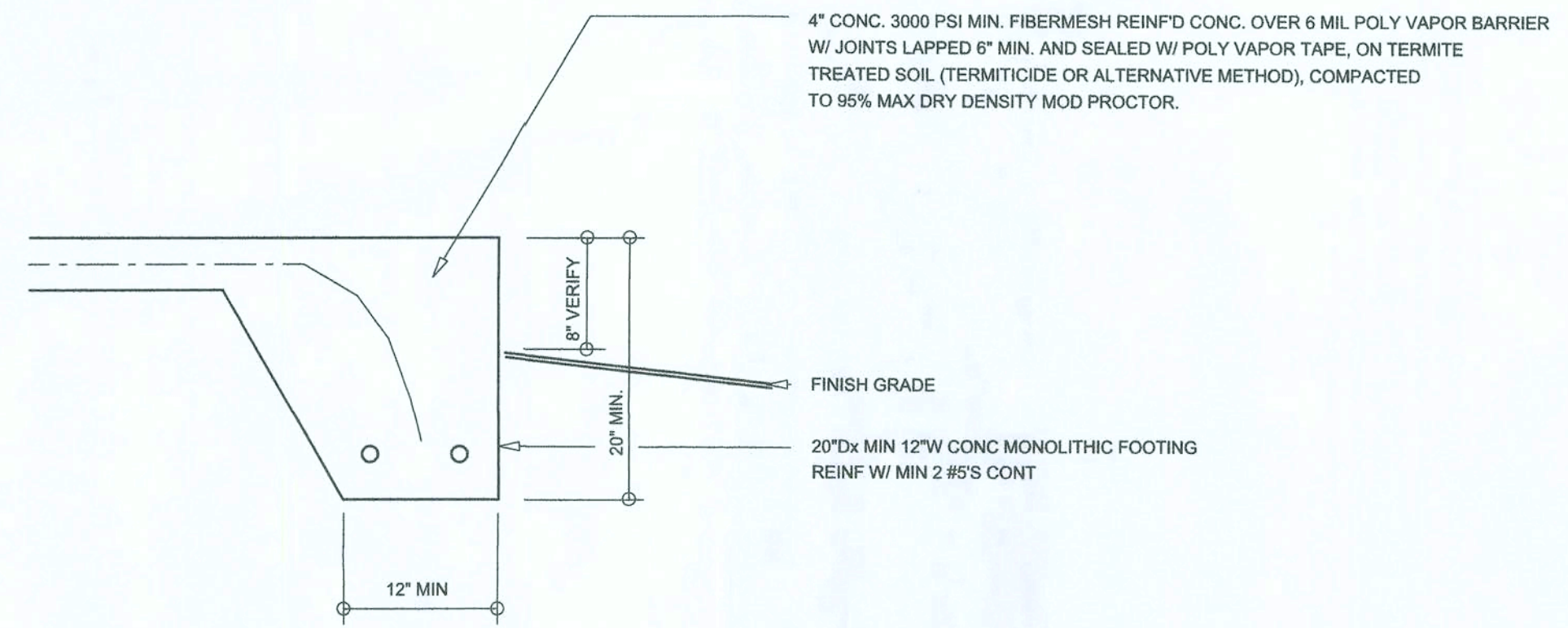
SECTION A SCALE: 3/4" = 1'-0" S.1
