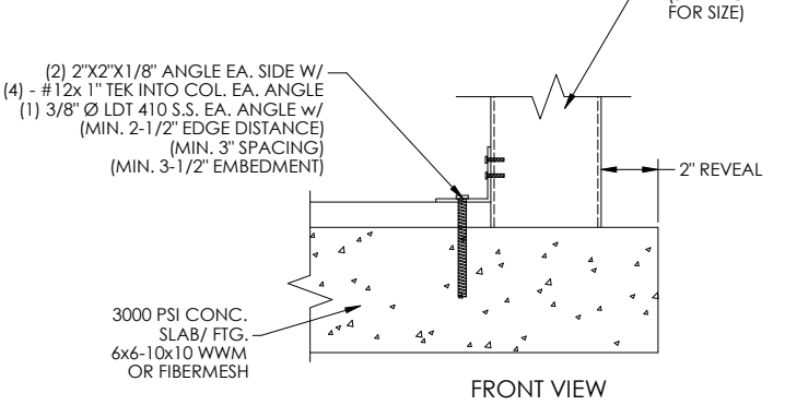
4"x4" POST CONNECTION DETAIL SCALE: N.T.S.
