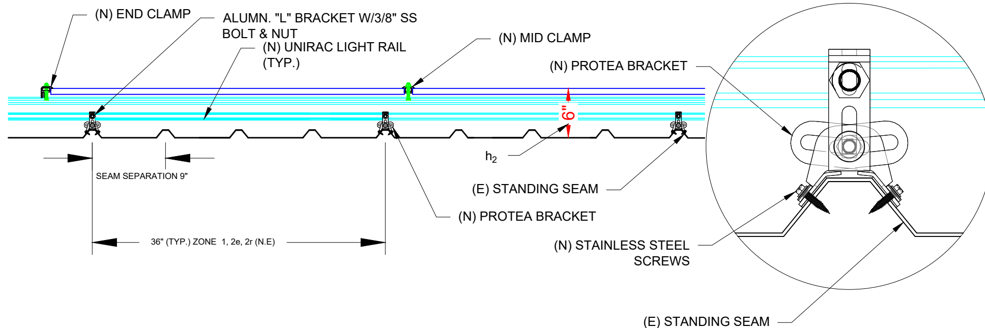
3 ENLARGE SECTION S-02 SCALE: NTS
