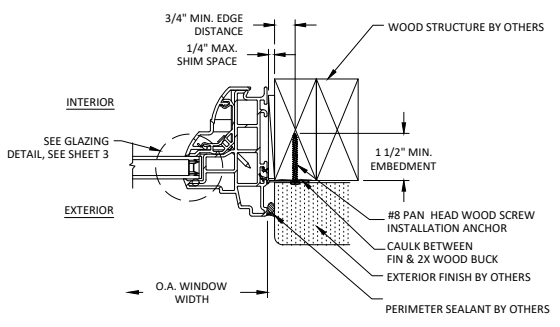
C 4 HORIZONTAL SECTION JAMB - WOOD BUCK NAIL FIN
