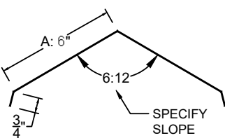
NOTCHABLE CAP (13.5")
