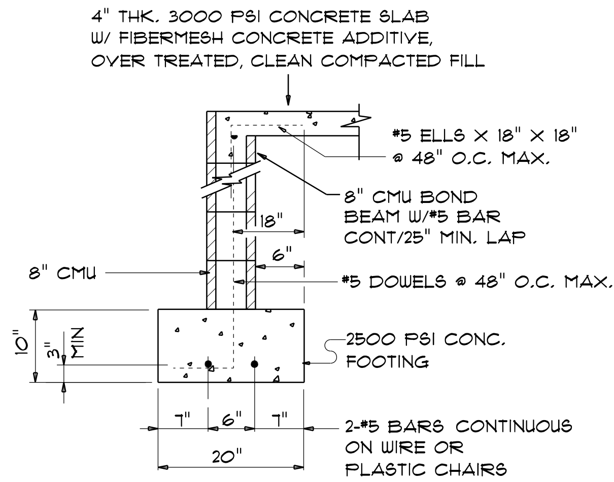
SECTION A SCALE: 3/4" = 1'-0" S.4
