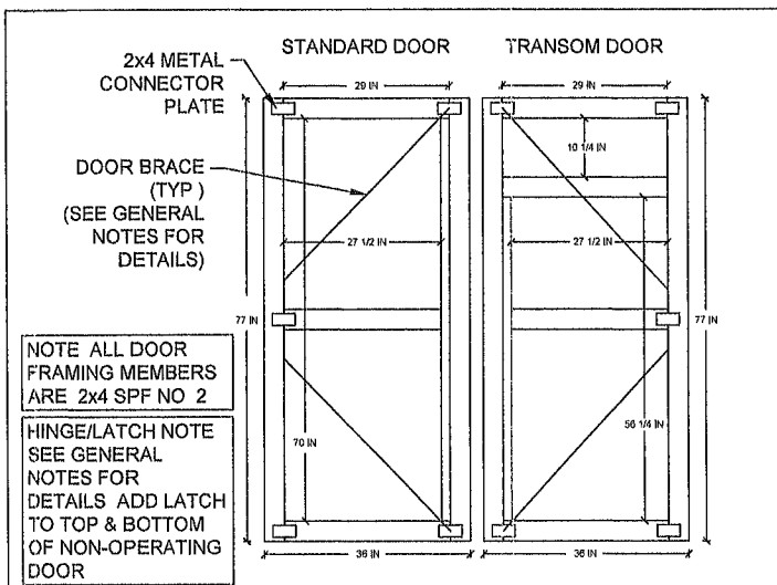
EXTERIOR DOOR DETAIL N.T.S.
