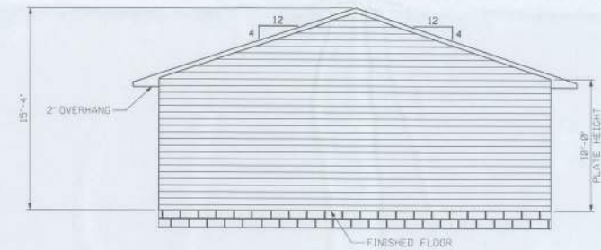
RIGHT ELEVATION
