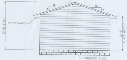
RIGHT ELEVATION
